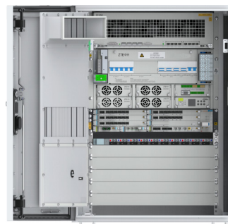
图 3-5 室外一体化 MEC
