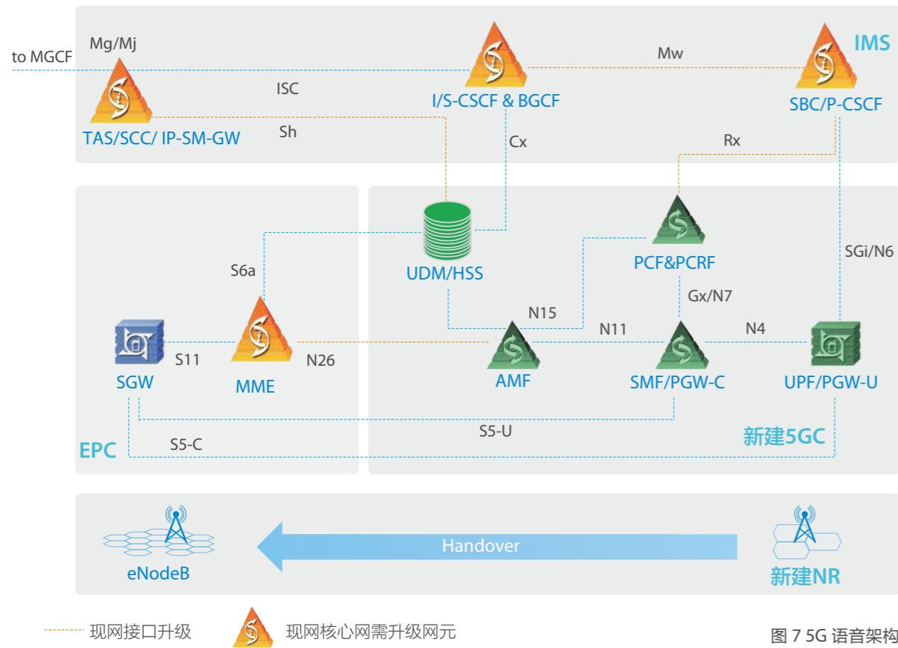
5G 语音体系架构如下图所示
